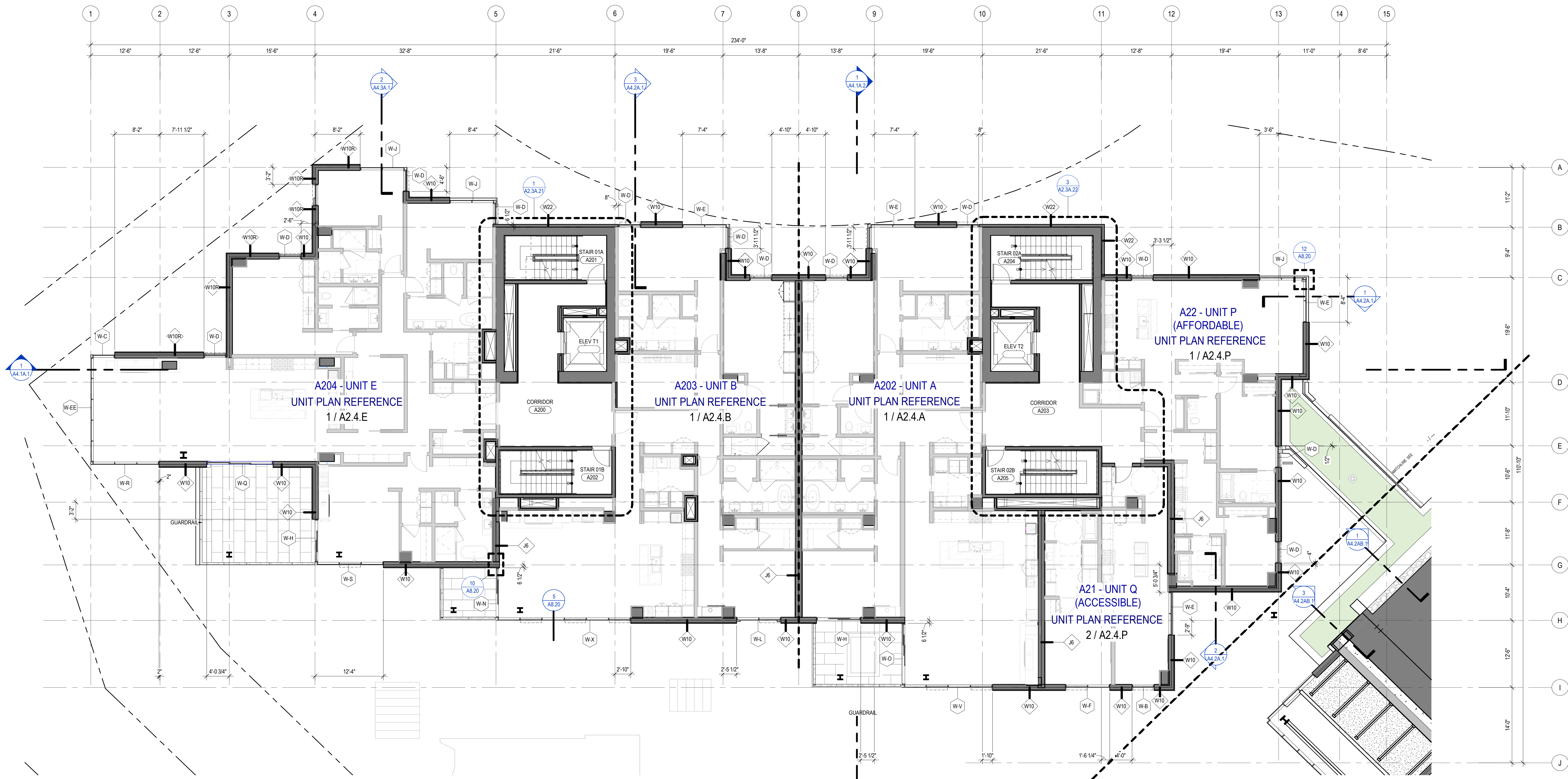
1 TOWER A - LEVEL 2 SCALE: 1/8" = 1'-0"
