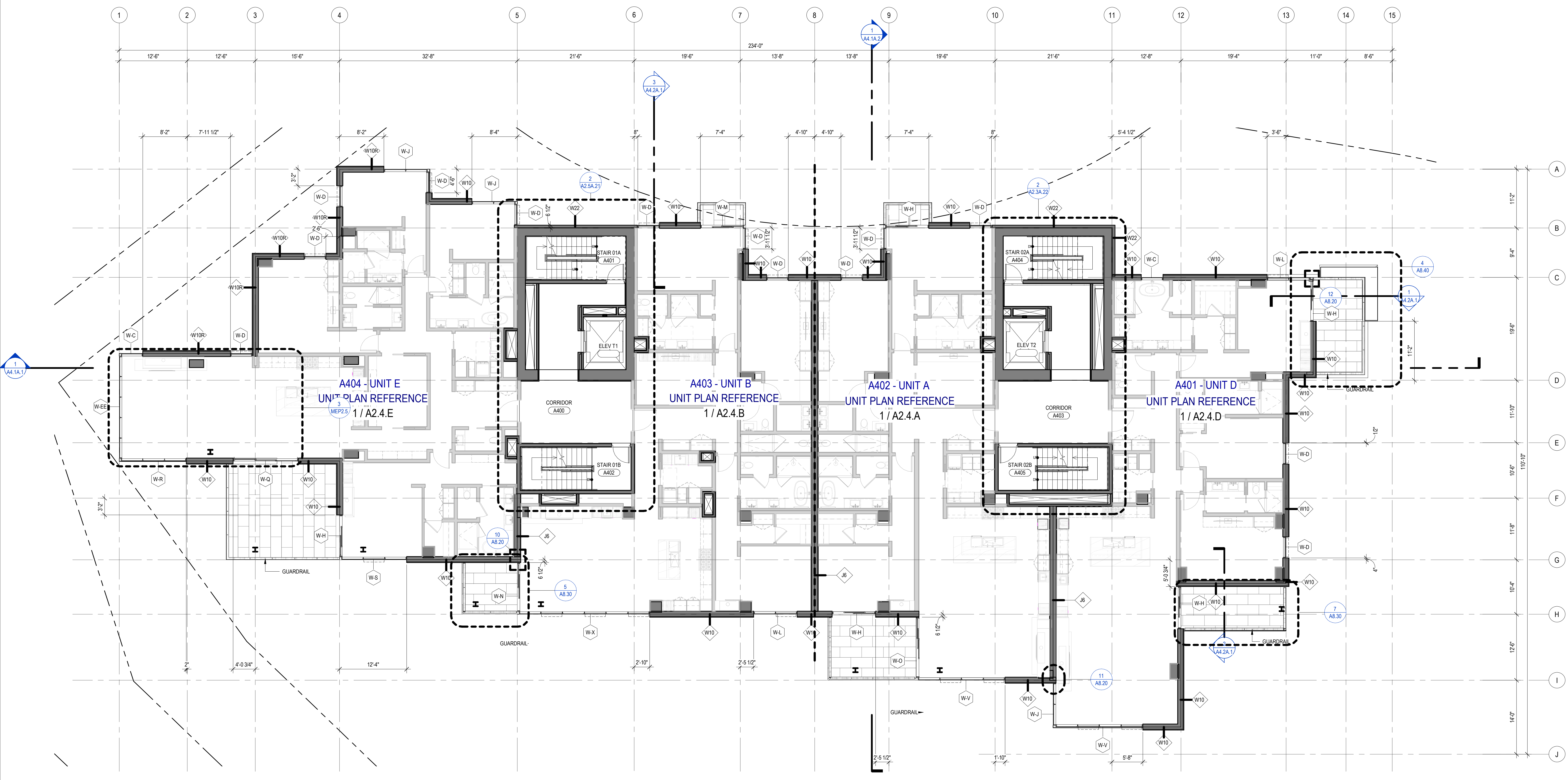
1 TOWER A - LEVEL 4 SCALE: 1/8" = 1'-0"
