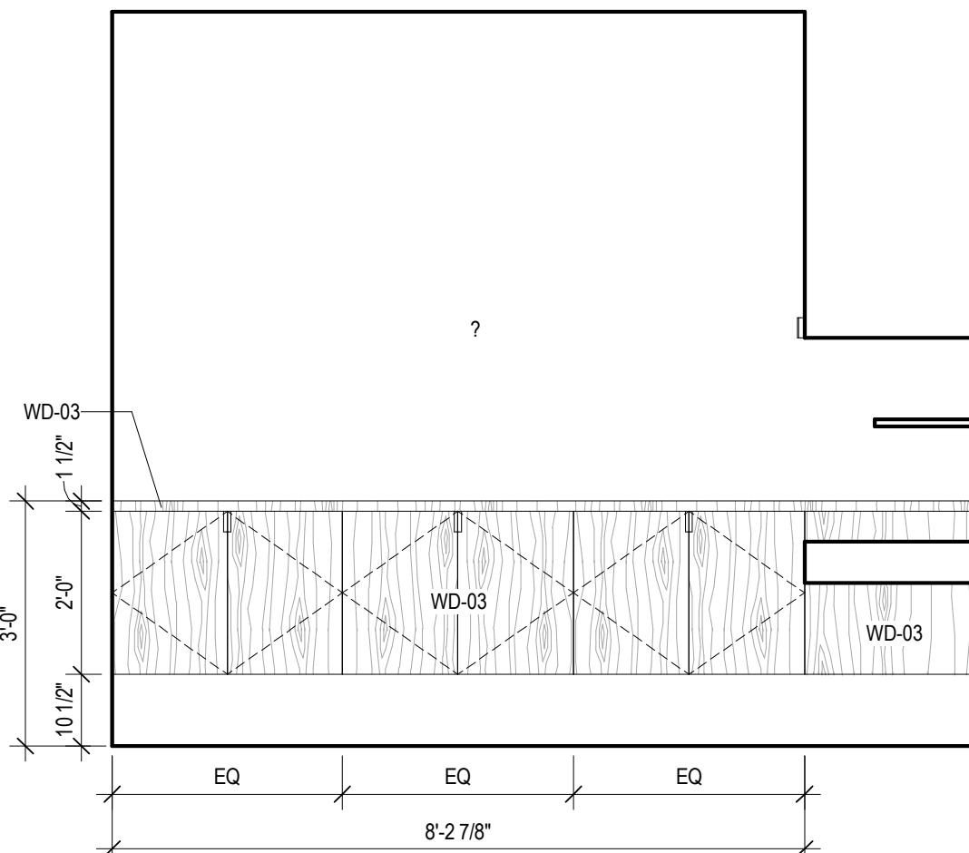
7 UNIT K - DEN CASEWORK - D SCALE: 1/2" = 1'-0"
