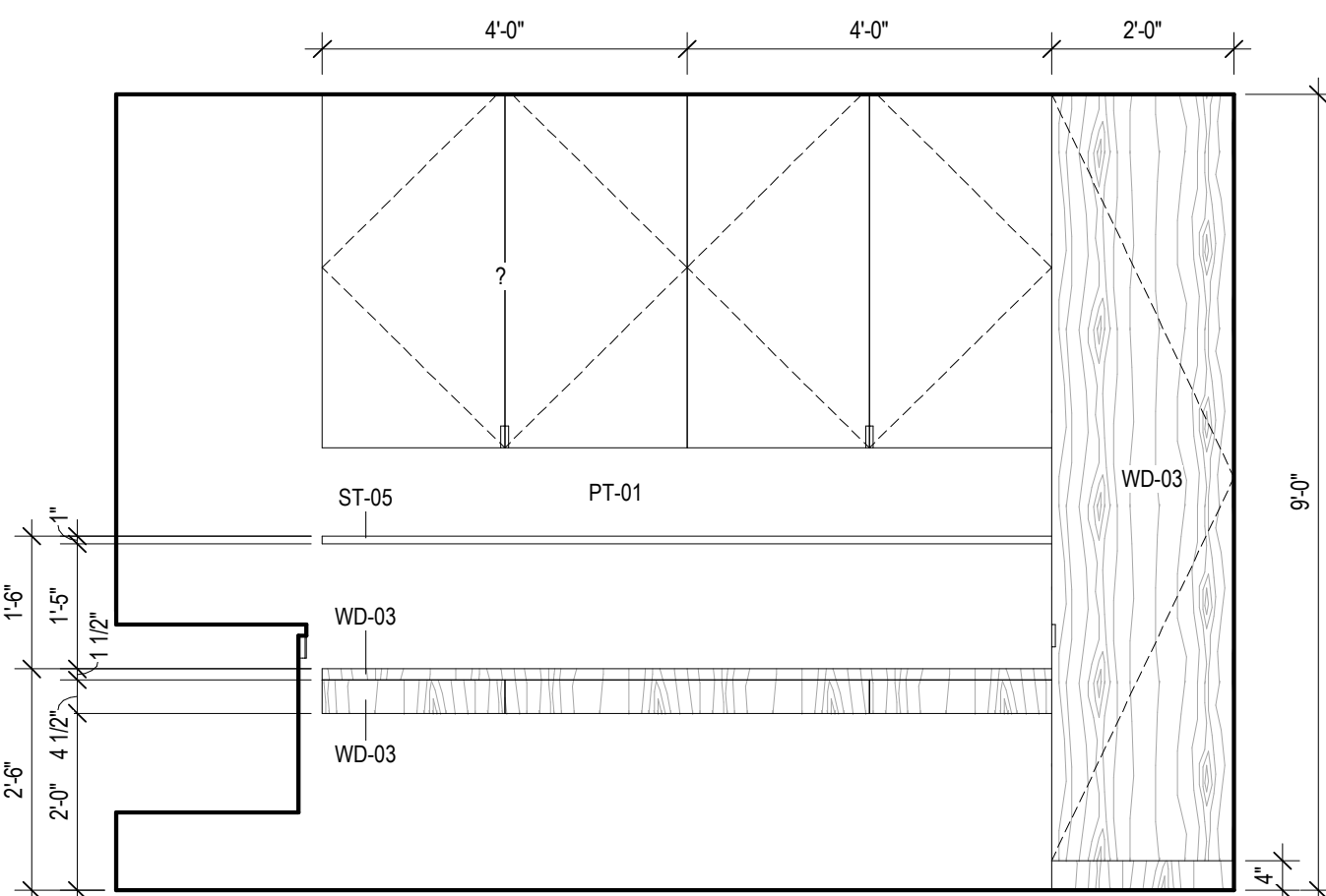
6 UNIT K - DEN CASEWORK - A SCALE: 1/2" = 1'-0"
