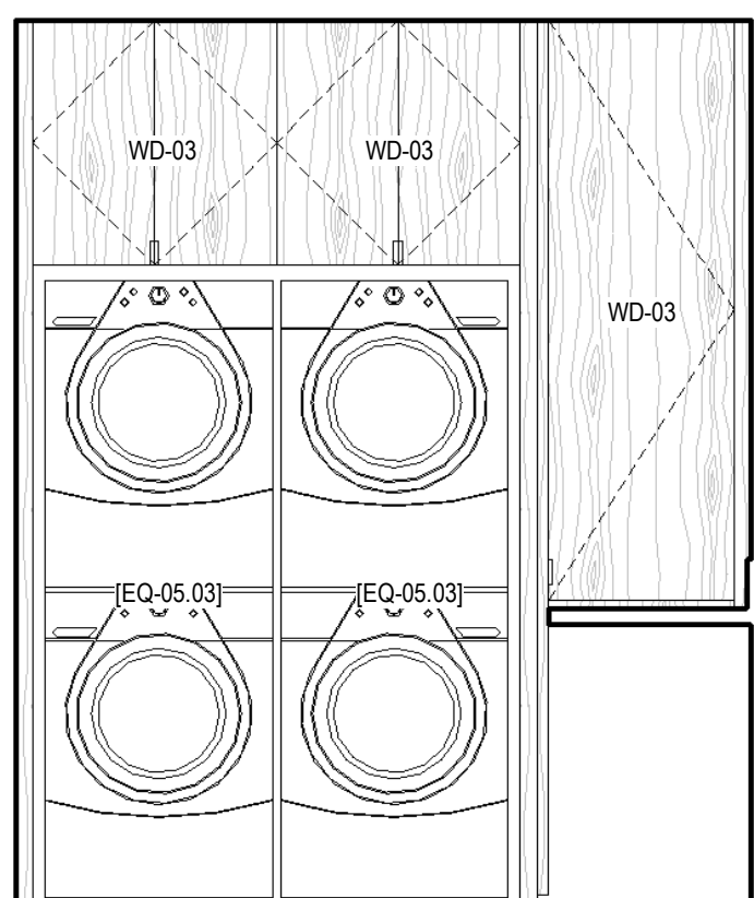
5 UNIT O - LAUNDRY - D SCALE: 1/2" = 1'-0"
