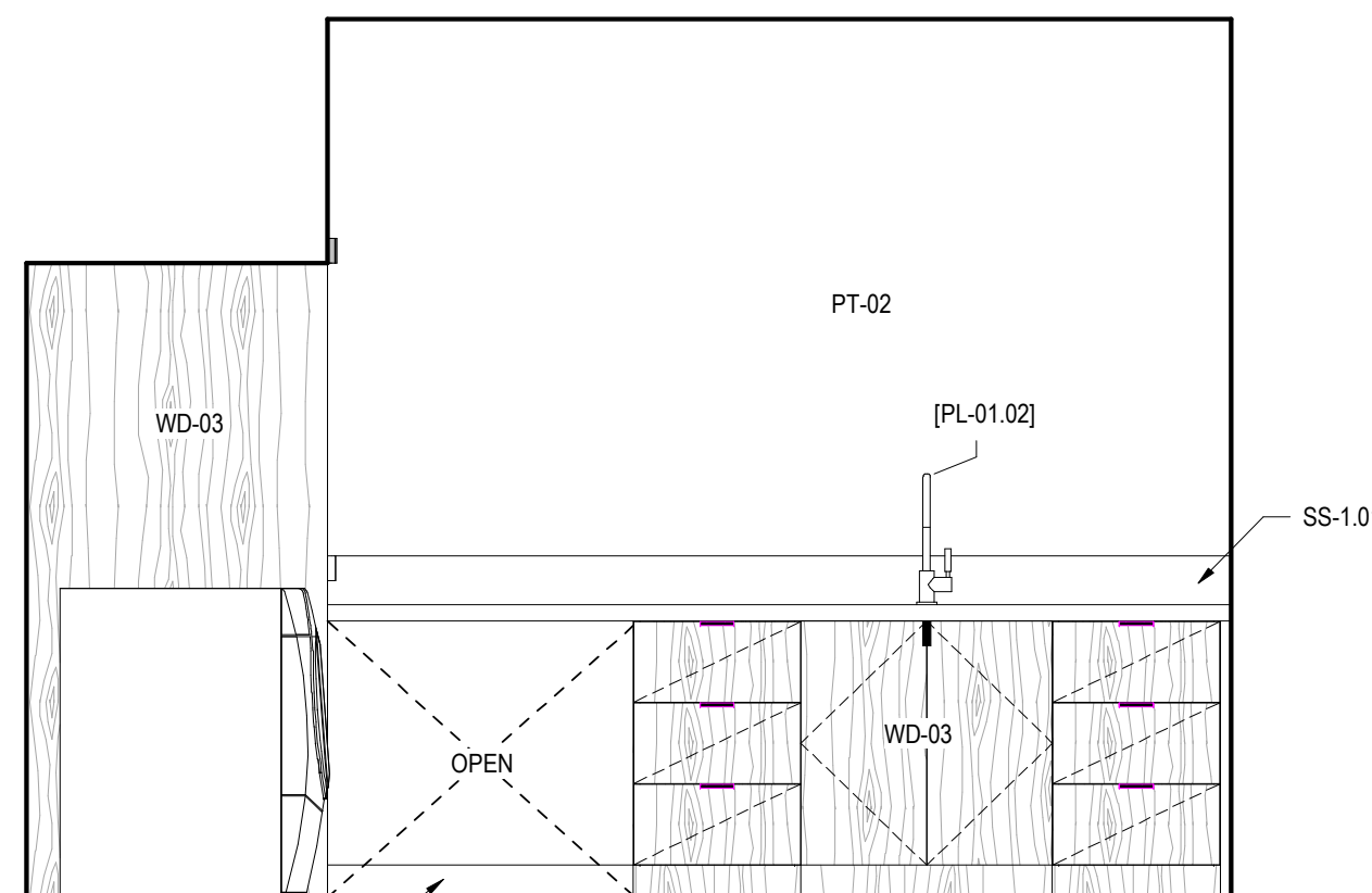
2 UNIT O - LAUNDRY - A SCALE: 1/2" = 1'-0"
