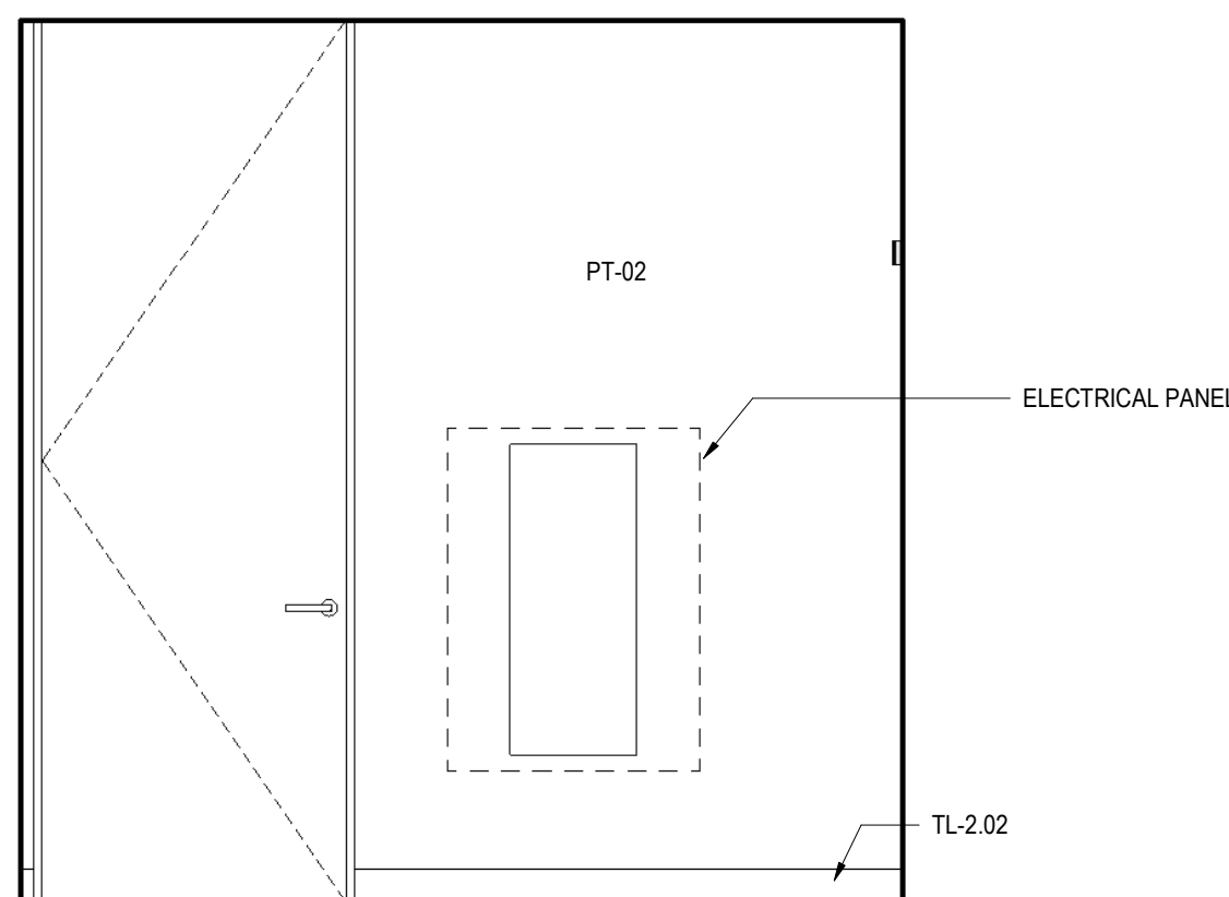
4 UNIT O - LAUNDRY - C SCALE: 1/2" = 1'-0"
