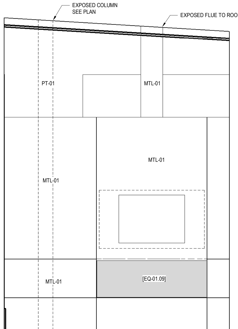
8 UNIT O - MASTER FP SCALE: 1/2" = 1'-0"
