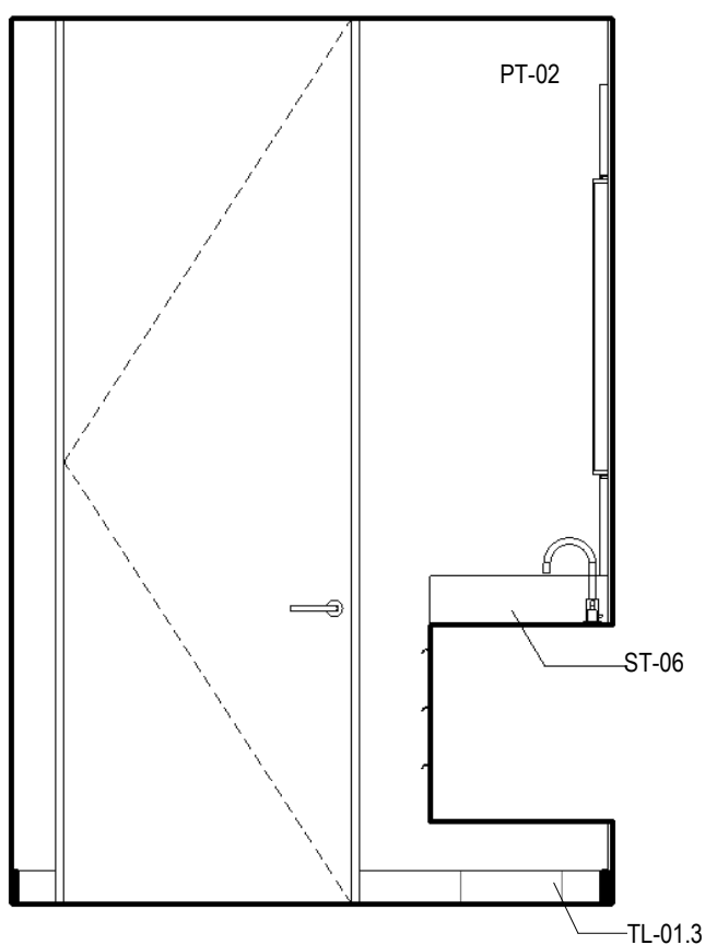
12 BATH ANSI A - LAYOUT 4 - D SCALE: 1/2" = 1'-0"
