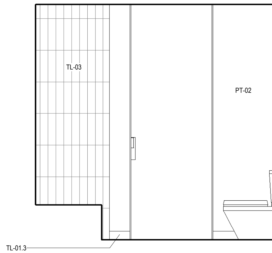
22 BATH ANSI B - LAYOUT 7 - TOILET B SCALE: 1/2" = 1'-0"
