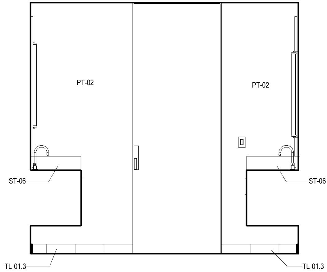
18 BATH ANSI B - LAYOUT 7 - B SCALE: 1/2" = 1'-0"
