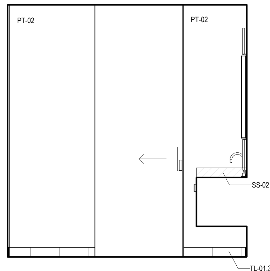
7 BATH ANSI A - LAYOUT 3 - B SCALE: 1/2" = 1'-0"
