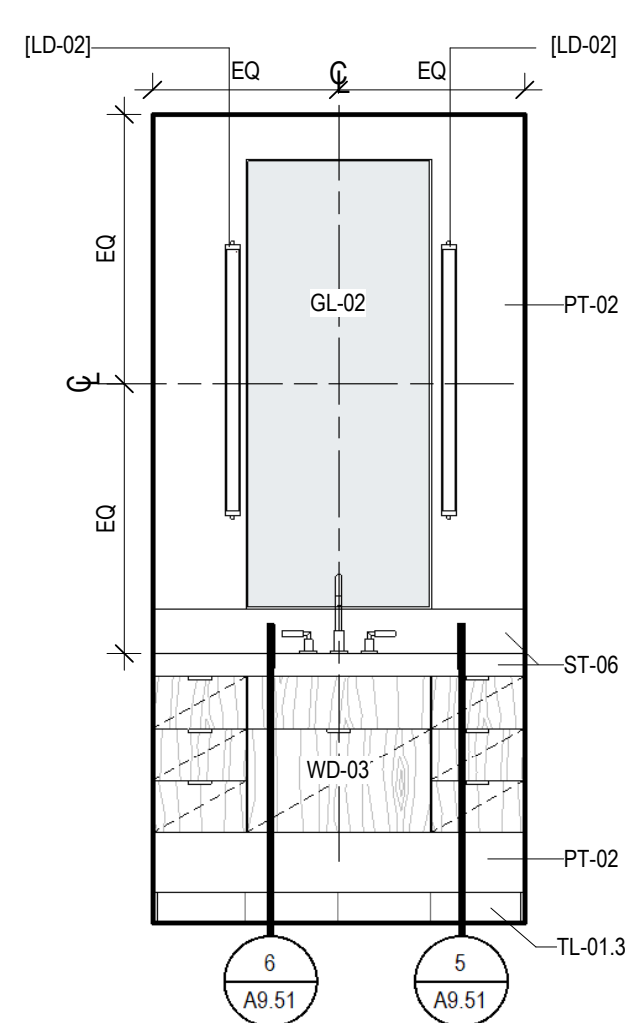
17 BATH ANSI B - LAYOUT 7 - A SCALE: 1/2" = 1'-0"
