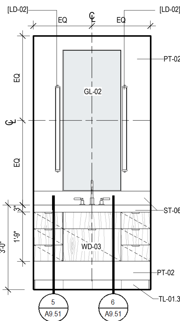
19 BATH ANSI B - LAYOUT 7 - C SCALE: 1/2" = 1'-0"
