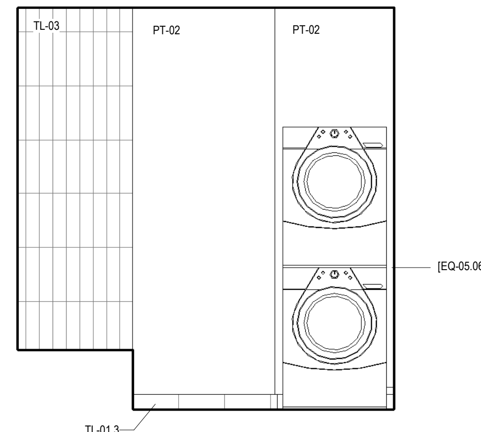
10 BATH ANSI A - LAYOUT 3 - A SCALE: 1/2" = 1'-0"
