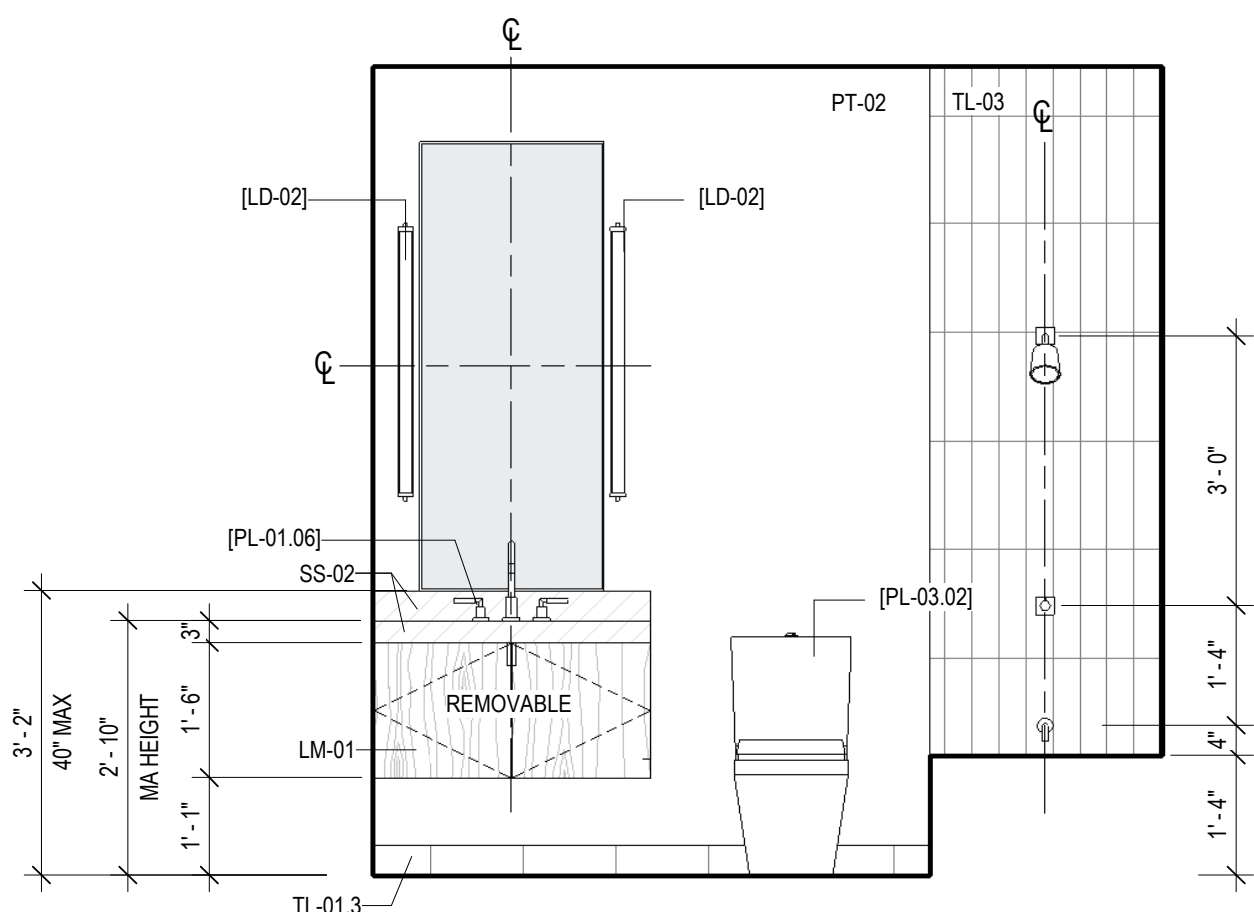
4 BATH ANSI A - LAYOUT 2 - C SCALE: 1/2" = 1'-0"
