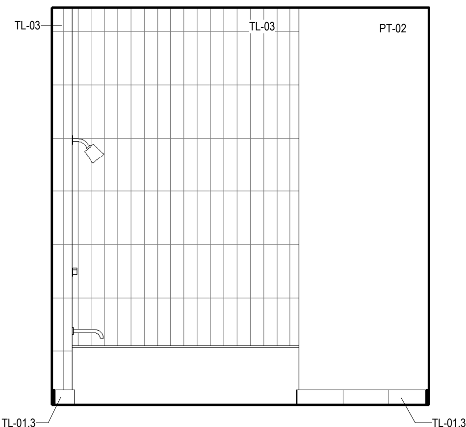
9 BATH ANSI A - LAYOUT 3 - D SCALE: 1/2" = 1'-0"
