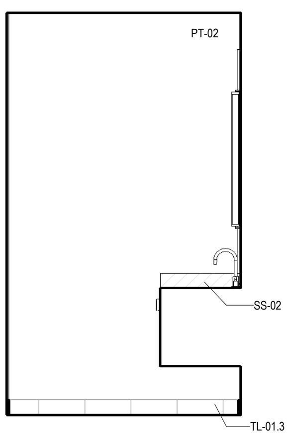
3 BATH ANSI A - LAYOUT 2 - B SCALE: 1/2" = 1'-0"
