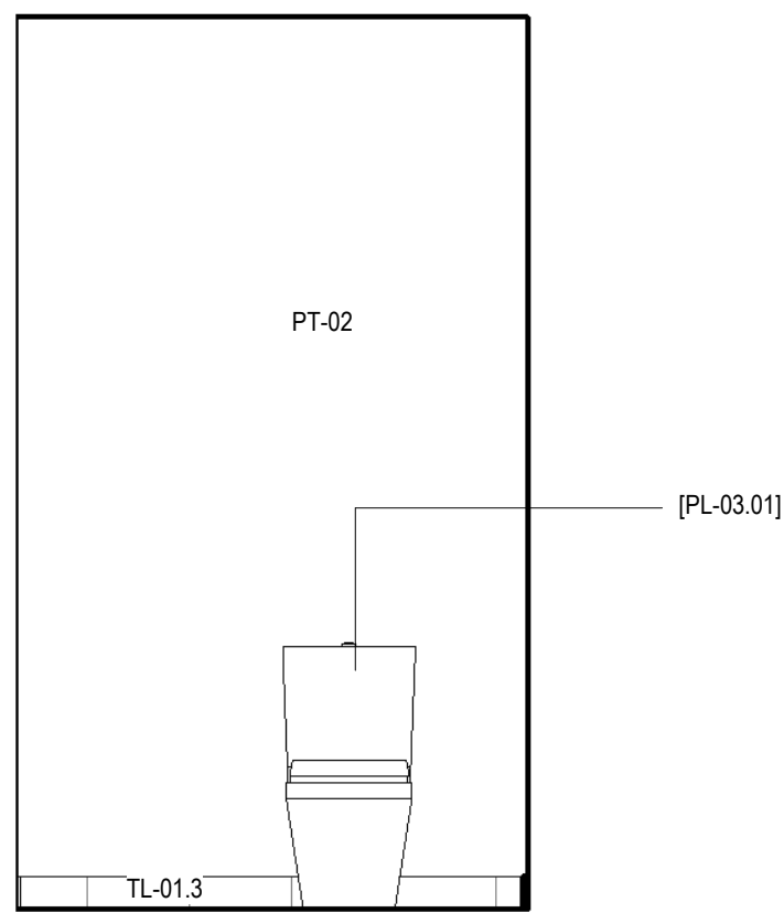
23 BATH ANSI B - LAYOUT 7 - TOILET C SCALE: 1/2" = 1'-0"
