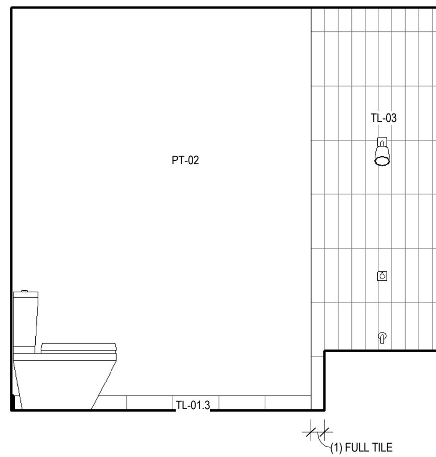
24 BATH ANSI B - LAYOUT 7 - TOILET D SCALE: 1/2" = 1'-0"
