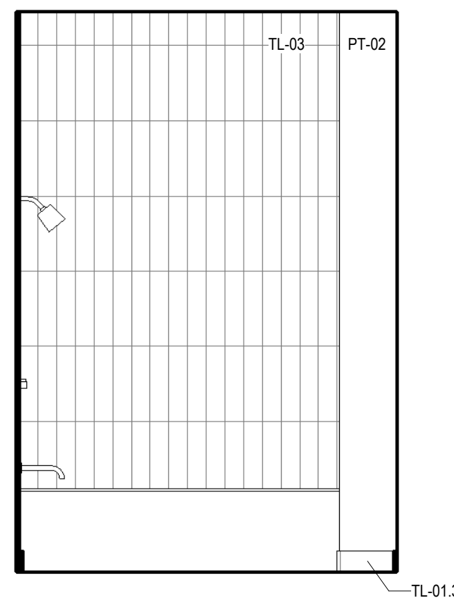
14 BATH ANSI A - LAYOUT 4 - B SCALE: 1/2" = 1'-0"
