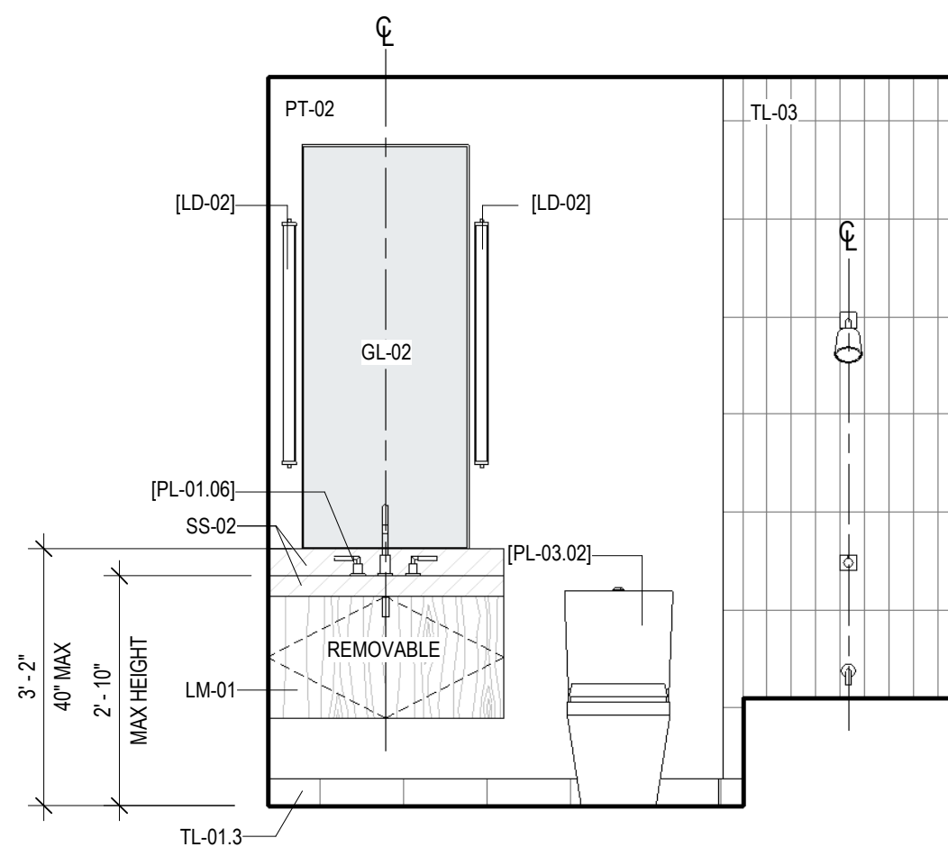
15 BATH ANSI A - LAYOUT 4 - C SCALE: 1/2" = 1'-0"
