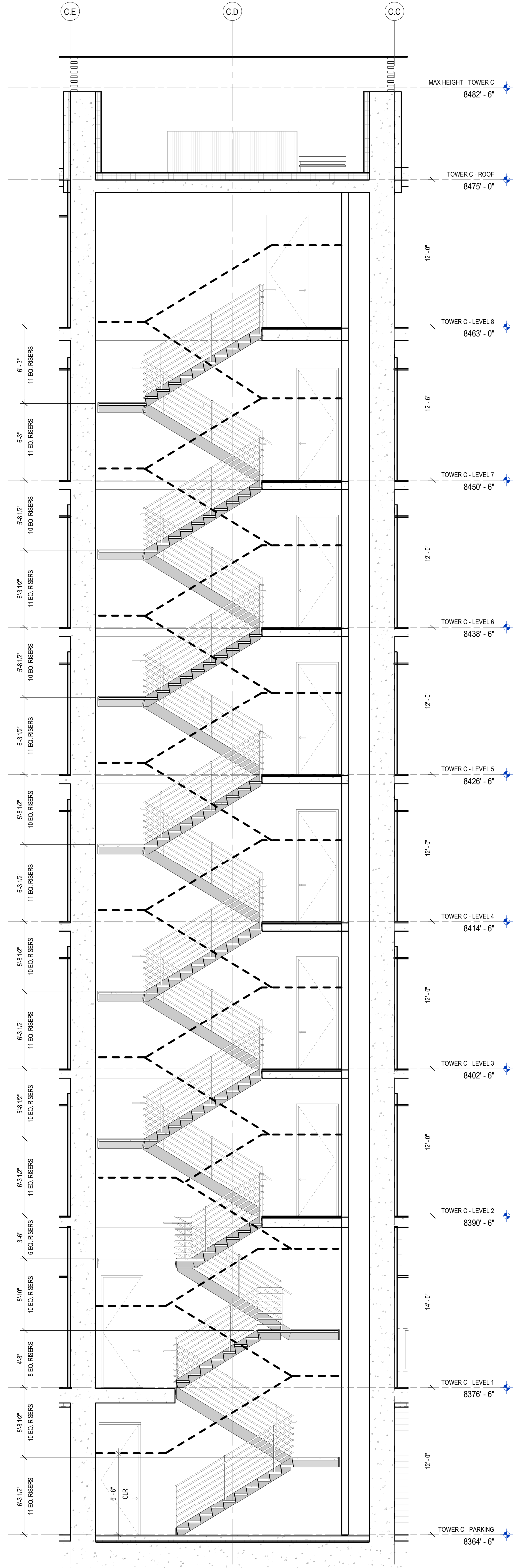
1 STAIR SECTION 1 - S05 SCALE: 1/4" = 1'-0"
