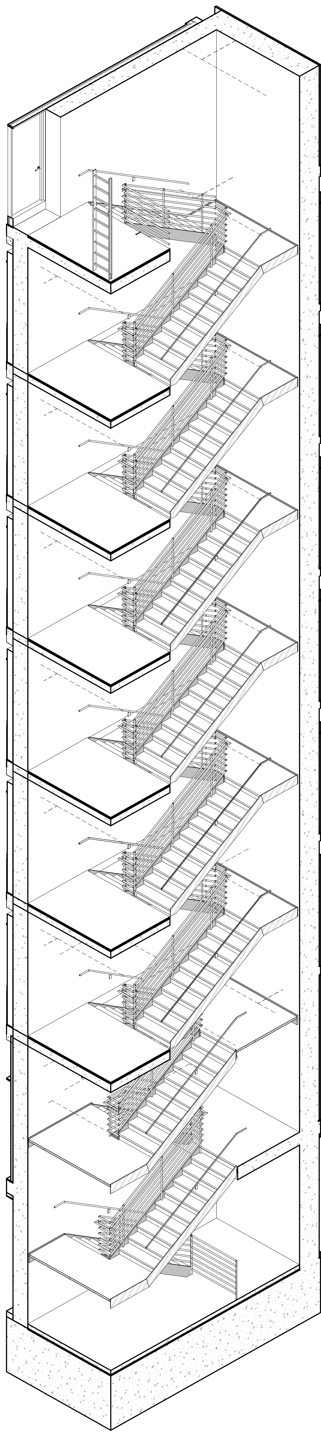
3 STAIR AXON - S05 SCALE: 1/4" = 1'-0"
