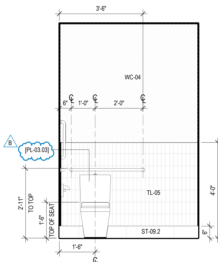
9 SPA TOILET, 188A - C SCALE: 1/2" = 1'-0"
