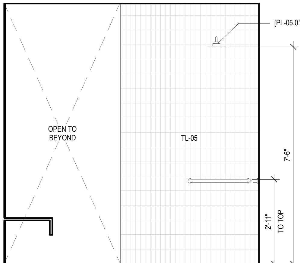
6 SPA TOILET, 188B - B SCALE: 1/2" = 1'-0"
