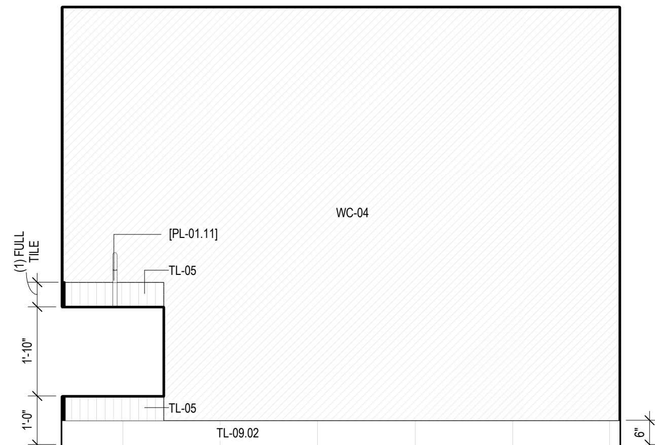
2 SPA TOILET, 188 - A SCALE: 1/2" = 1'-0"
