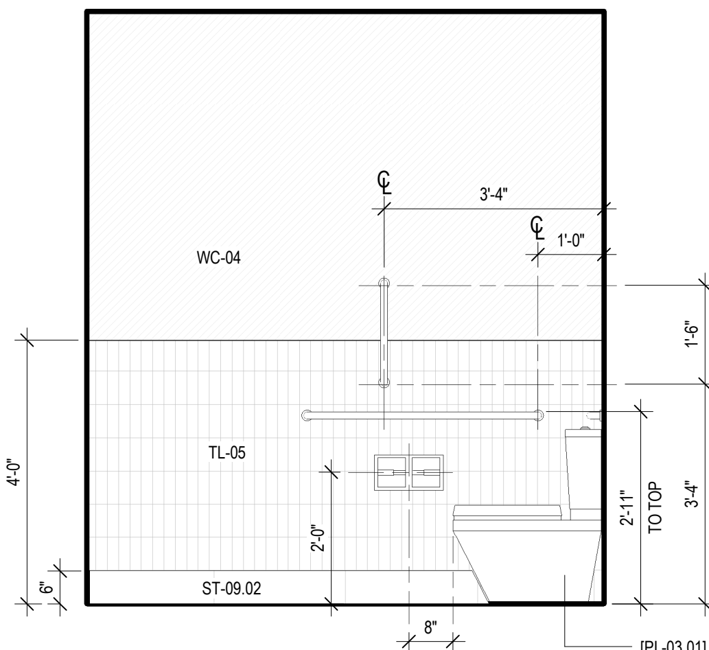
10 SPA TOILET, 188A - D SCALE: 1/2" = 1'-0"
