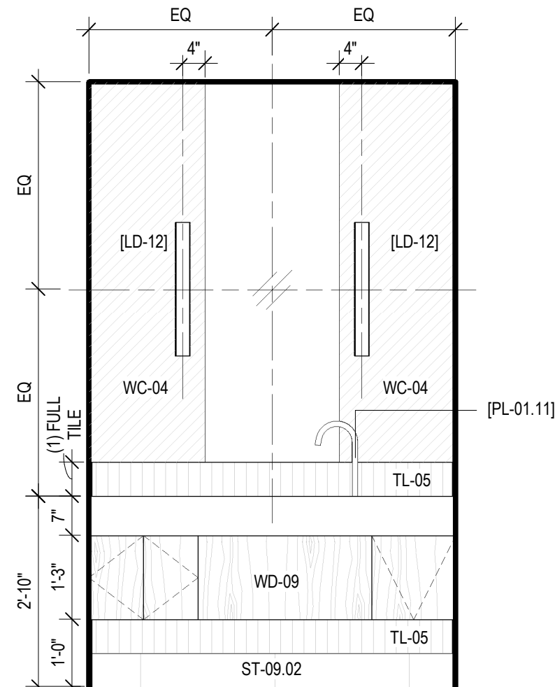
3 SPA TOILET, 188 - B SCALE: 1/2" = 1'-0"
