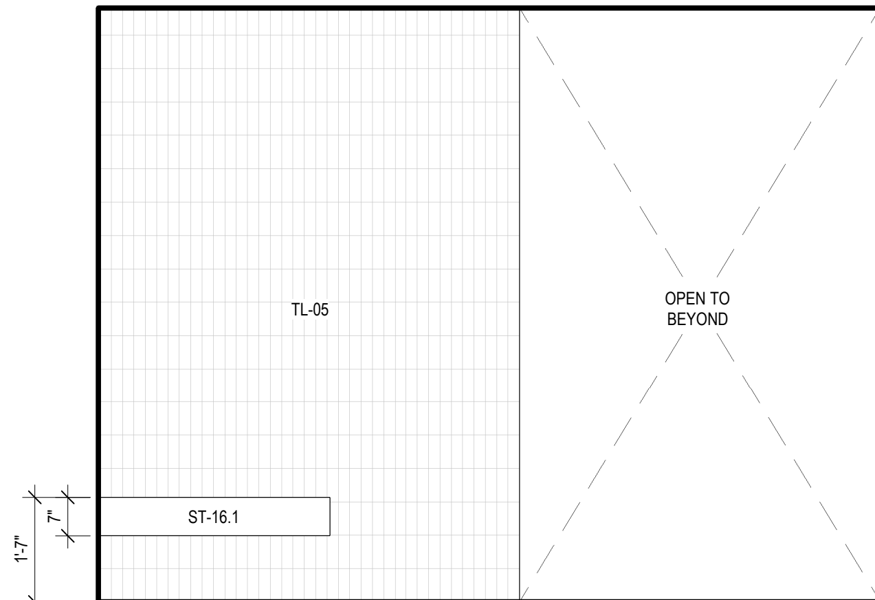
7 SPA TOILET, 188B - C SCALE: 1/2" = 1'-0"
