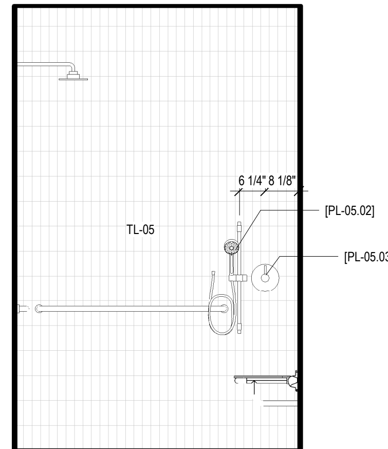
5 SPA TOILET, 188B - A SCALE: 1/2" = 1'-0"
