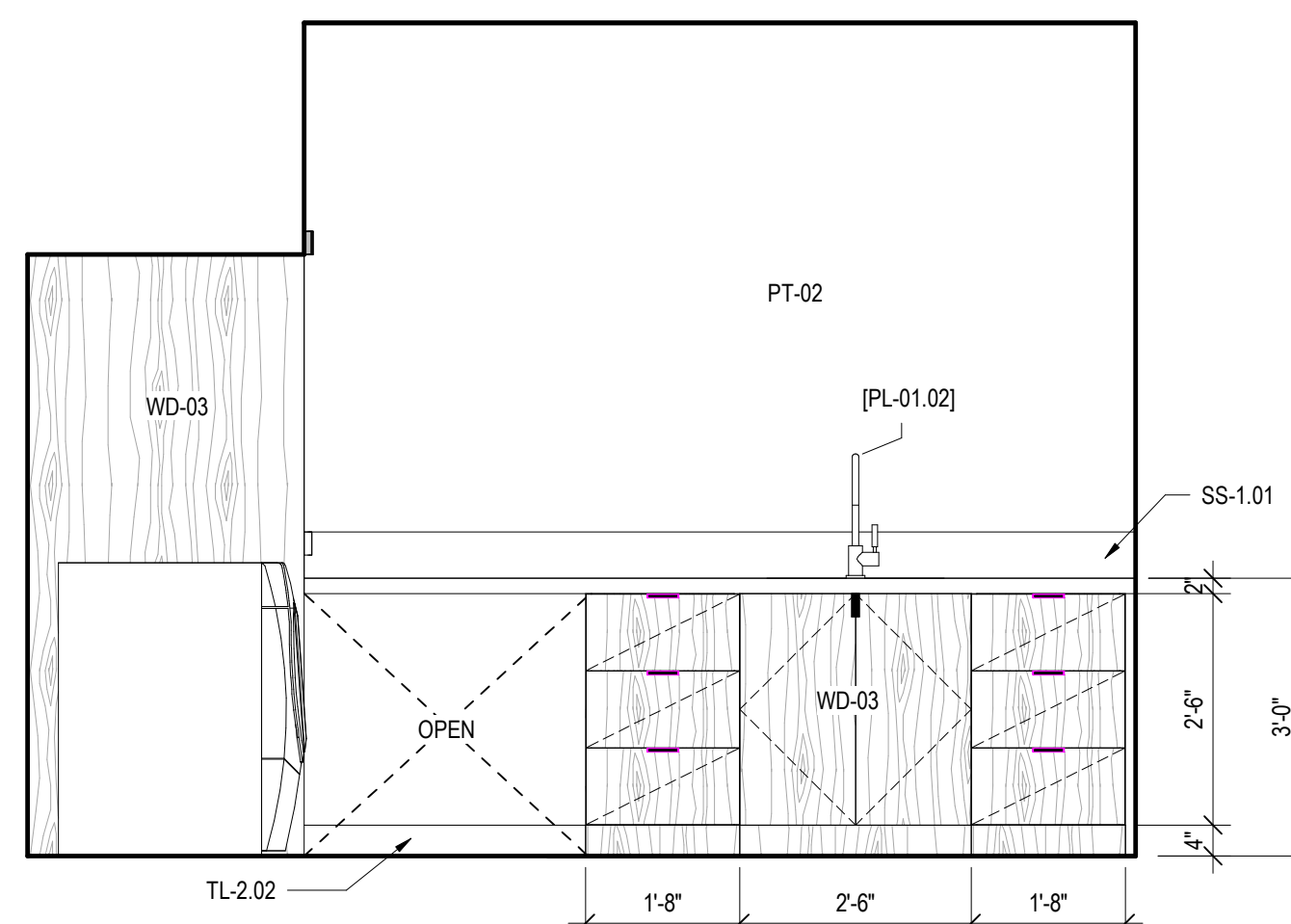
2 UNIT O - LAUNDRY - A SCALE: 1/2" = 1'-0"
