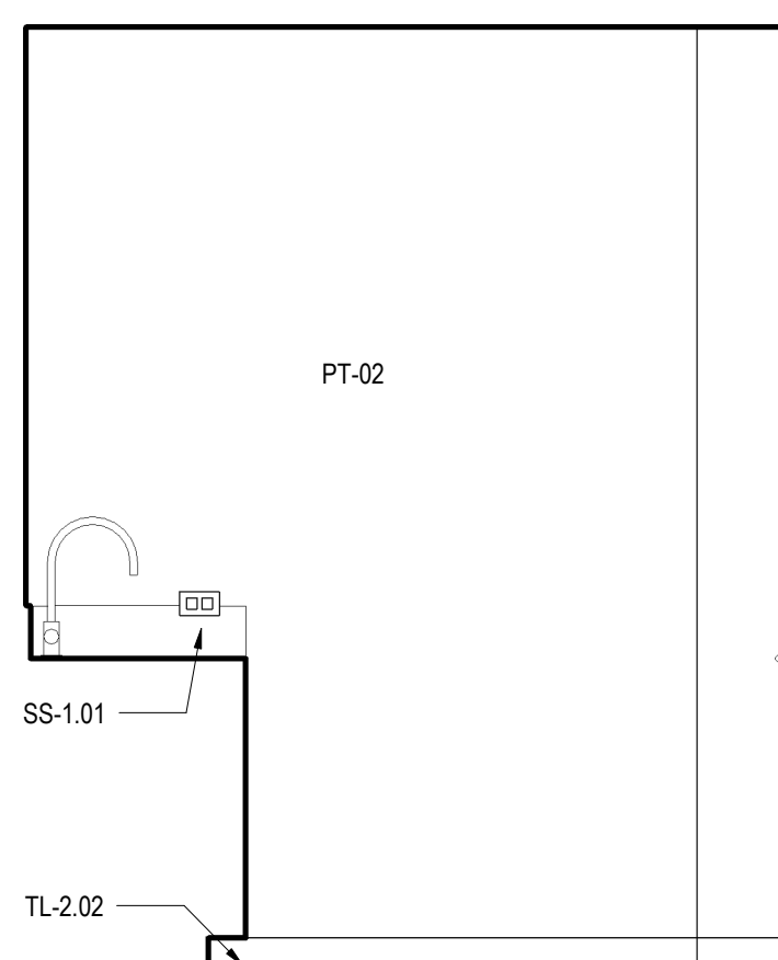
3 UNIT O - LAUNDRY - B SCALE: 1/2" = 1'-0"
