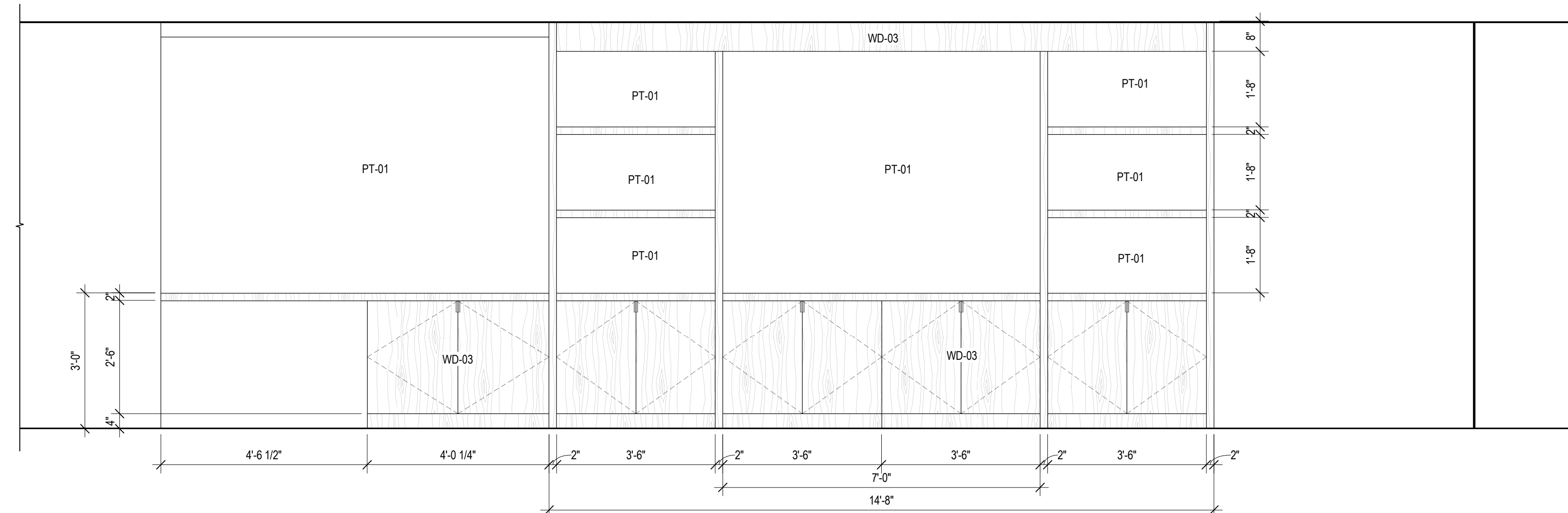
7 UNIT O - CORRIDOR - A SCALE: 1/2" = 1'-0"
