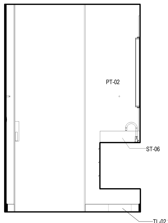
16 BATH 9 - D SCALE: 1/2" = 1'-0"
