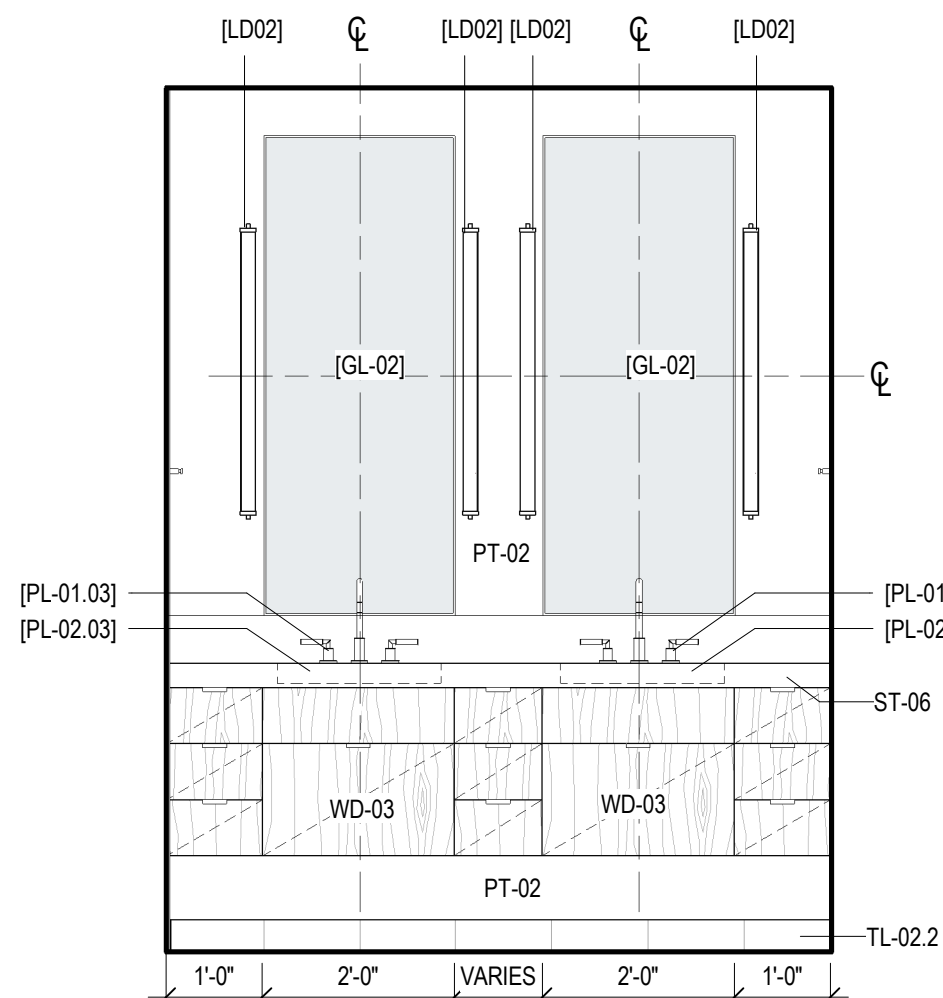
13 BATH 9 - A SCALE: 1/2" = 1'-0"
