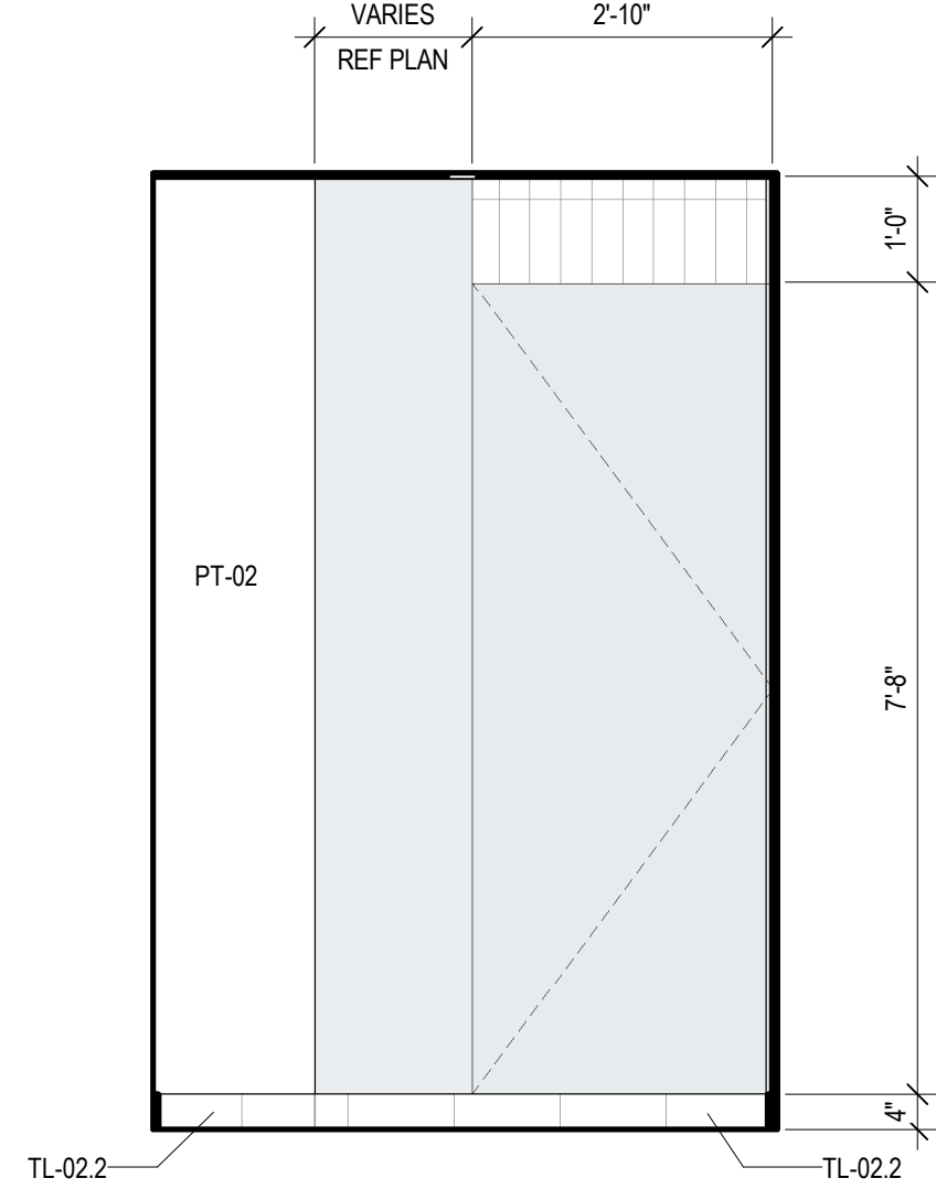
21 BATH 9 - TOILET B SCALE: 1/2" = 1'-0"
