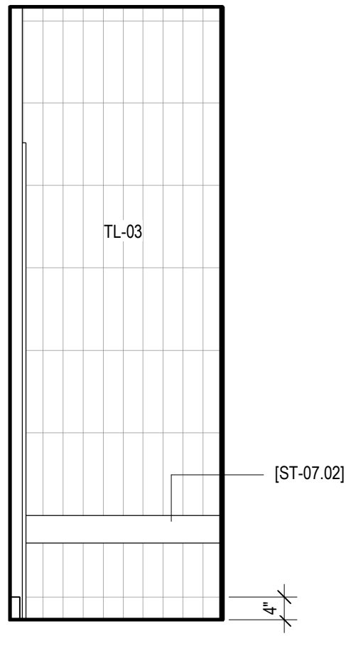
17 BATH 9 - SHOWER A SCALE: 1/2" = 1'-0"
