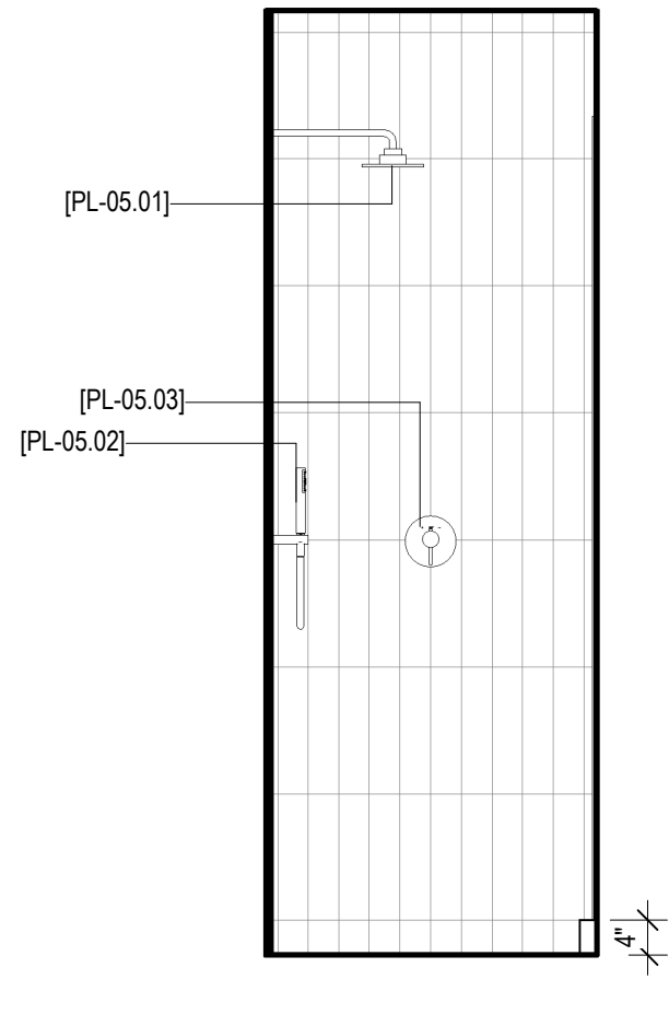
19 BATH 9 - SHOWER C SCALE: 1/2" = 1'-0"
