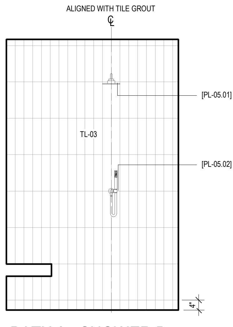
18 BATH 9 - SHOWER B SCALE: 1/2" = 1'-0"
