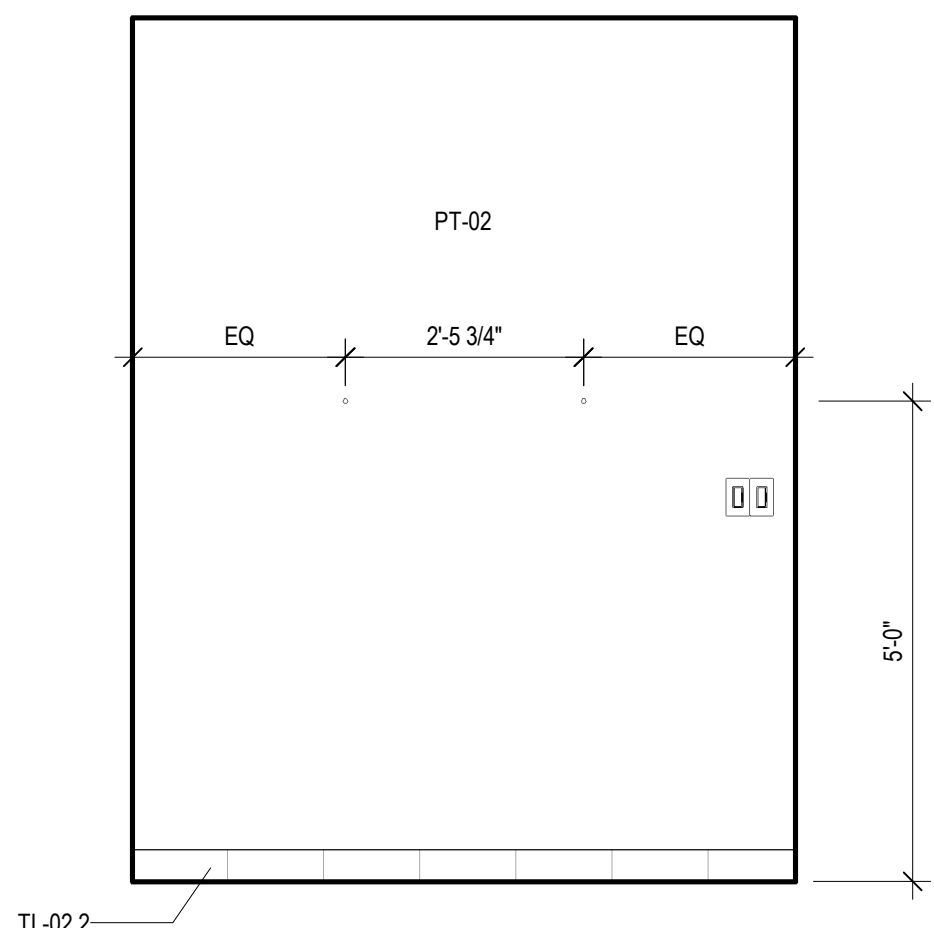
15 BATH 9 - C SCALE: 1/2" = 1'-0"
