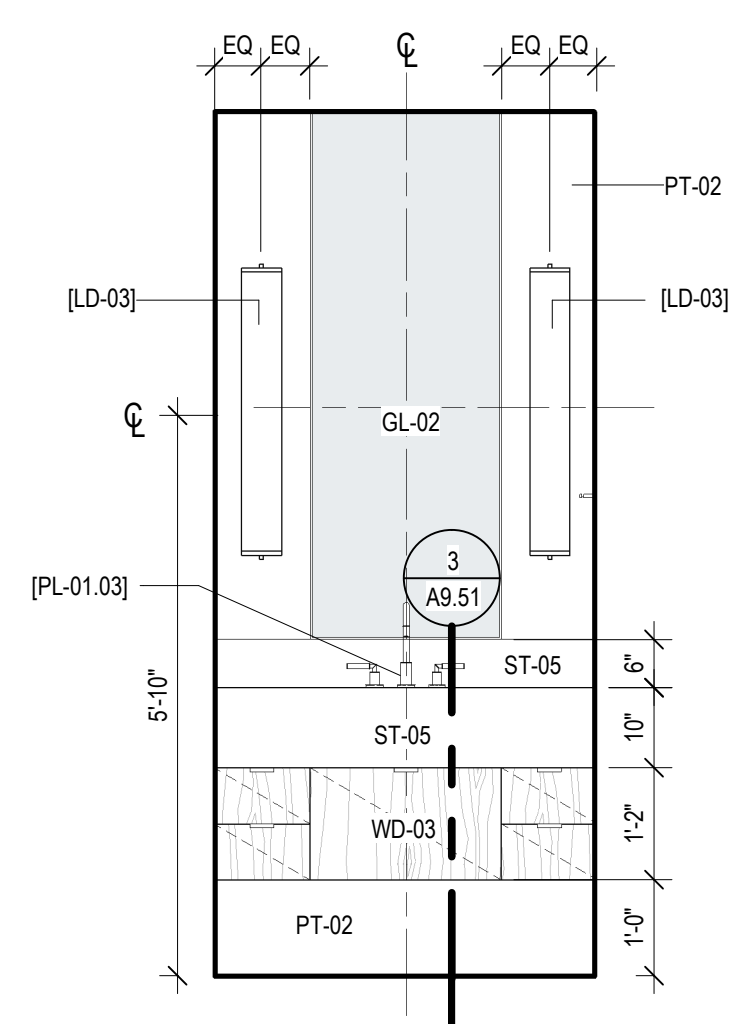
10 POWDER 2 - D SCALE: 1/2" = 1'-0"
