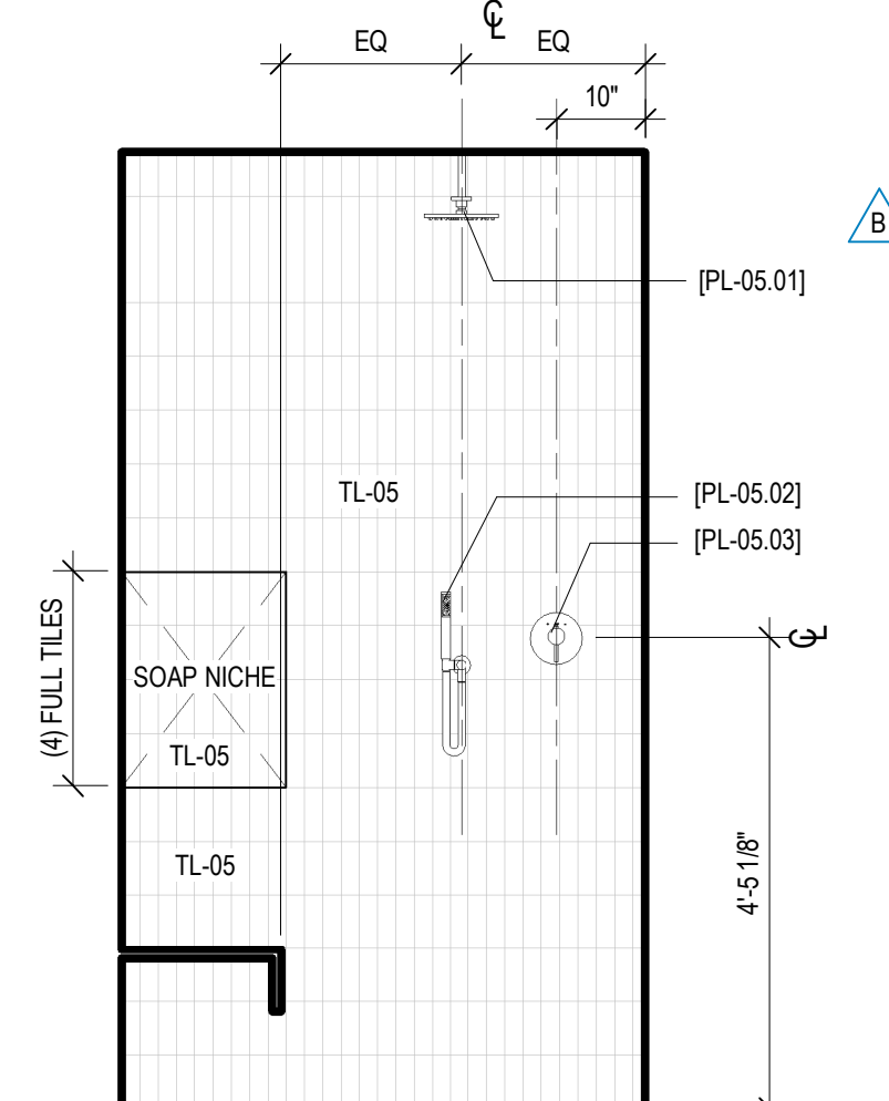
6 SPA TOILET, 606B - A SCALE: 1/2" = 1'-0"
