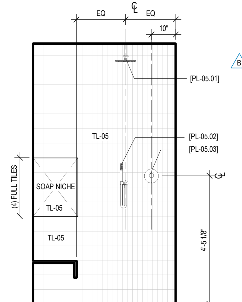
6 SPA TOILET, 606B - A SCALE: 1/2" = 1'-0"
