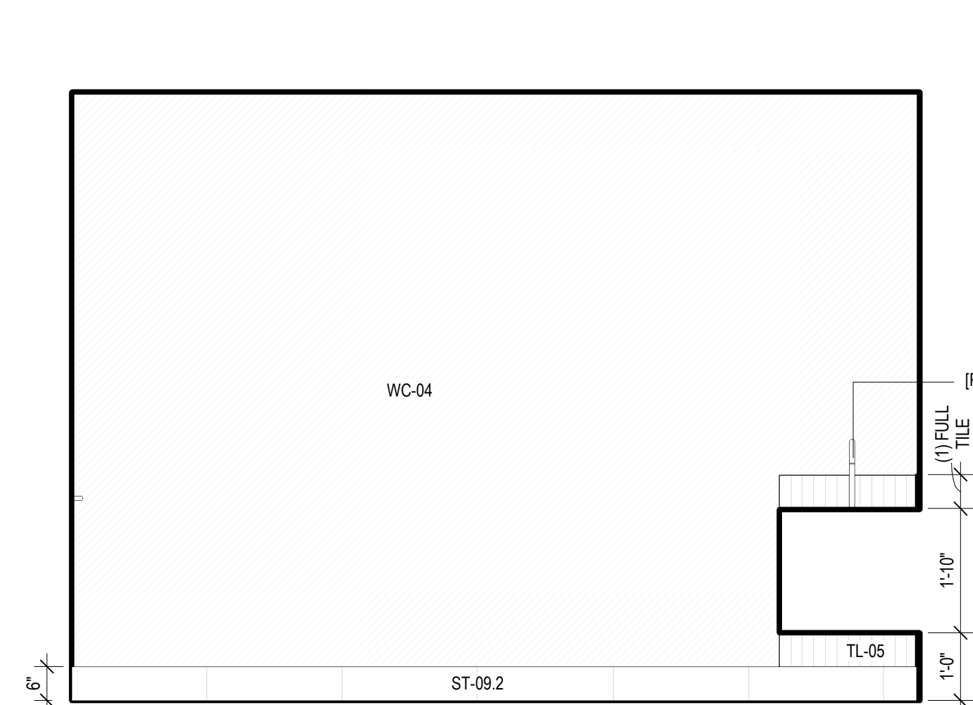
13 SPA TOILET, 606 - D SCALE: 1/2" = 1'-0"
