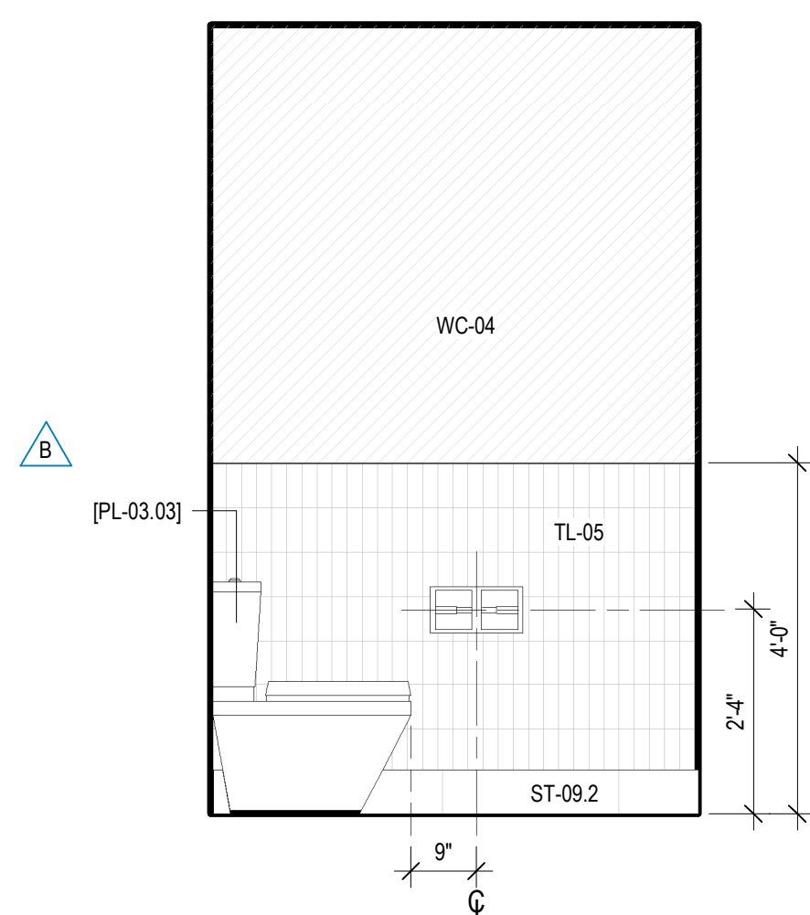
3 SPA TOILET, 606A - B SCALE: 1/2" = 1'-0"
