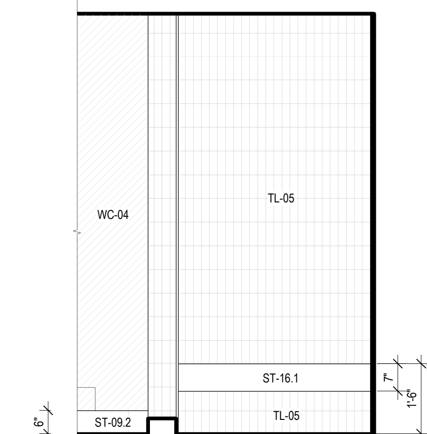
7 SPA TOILET, 606 - F SCALE: 1/2" = 1'-0"
