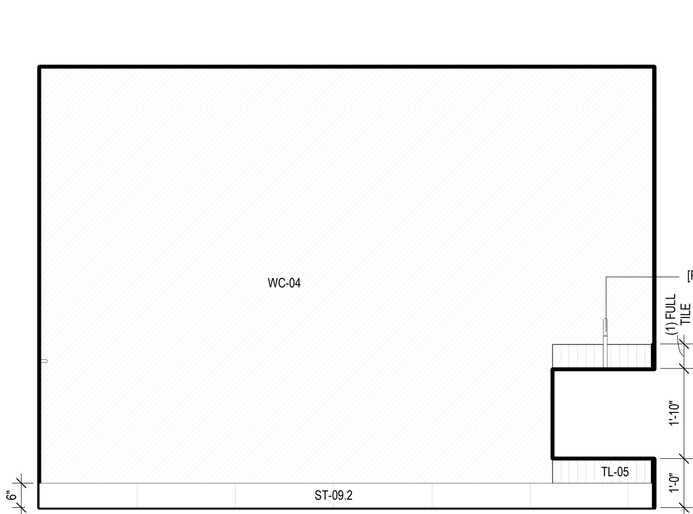
13 SPA TOILET, 606 - D SCALE: 1/2" = 1'-0"
